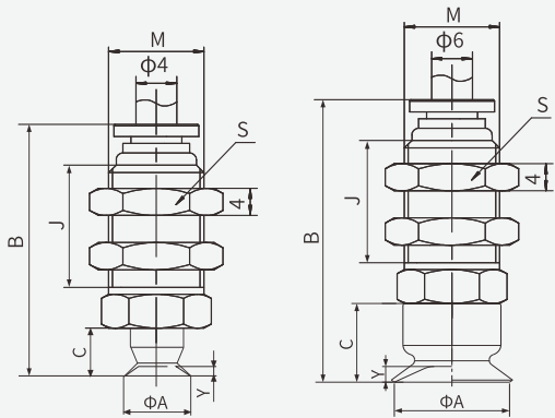
适合吸盘直径15-20
