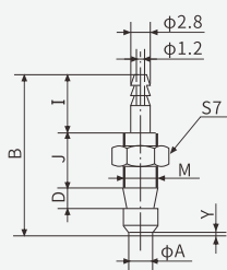
垂直方向-宝塔接头
