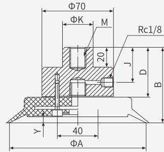
适合吸盘直径120-200
