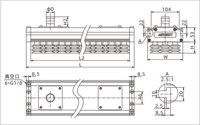
TXM130×400(600-1400)-B 吸盘型
