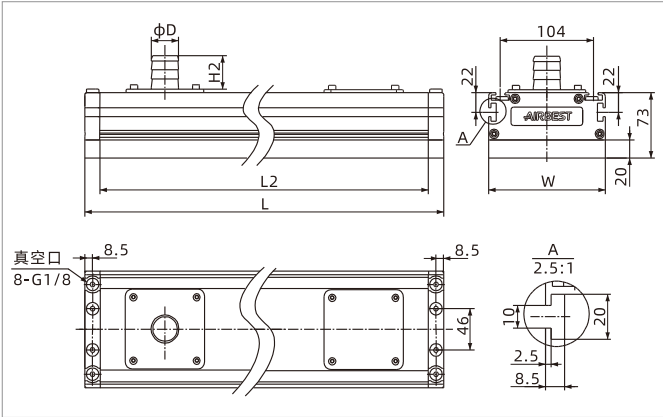
TXM130×400(600-1400)-A 海绵型
