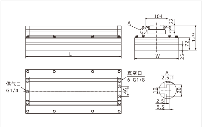
TXL 海绵型
