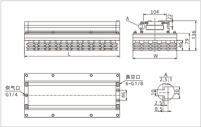
TXL 吸盘型
