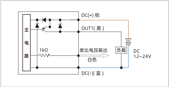
ZPDT-CPV-R1M 1PNP+类比电压输出（1-5V）
