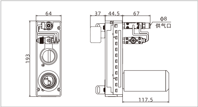
AMC25□-□-V-ES AMC50□-□-V-ES
