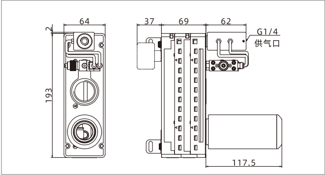
AMC75□-□-V-ES AMC100□-□-V-ES
