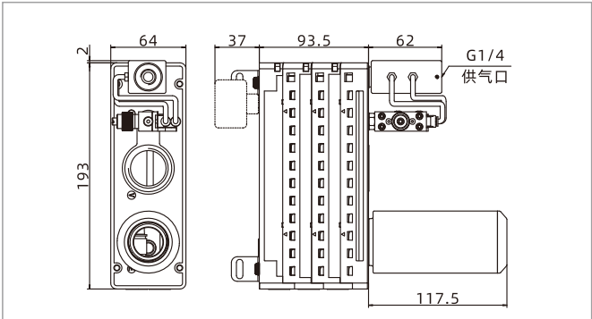
AMC125□-□-V-ES AMC150□-□-V-ES
