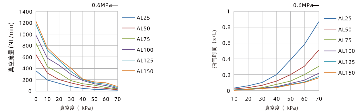
AH系列不同真空度（-kPa）的真空流量（NL/min）
