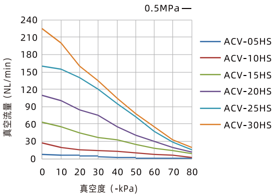
不同真空度（-kPa）的真空流量（NL/min）
