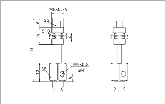
SP3C4-16 水平可回转 SP3C4-16 水平不可回转
