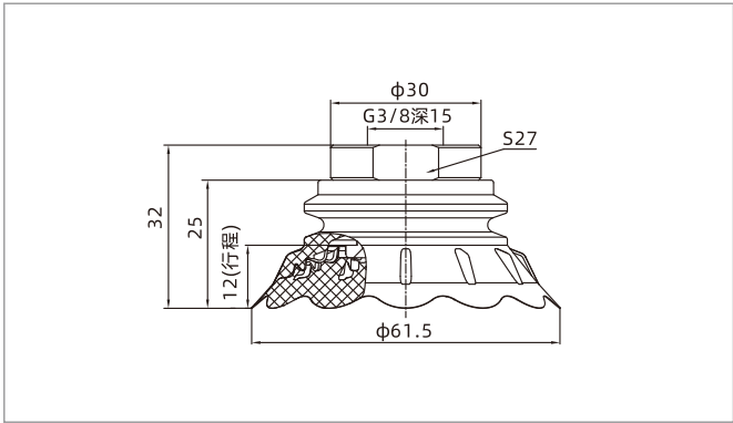
STP60□-G3F
