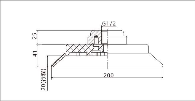
SF200 内螺纹连接
