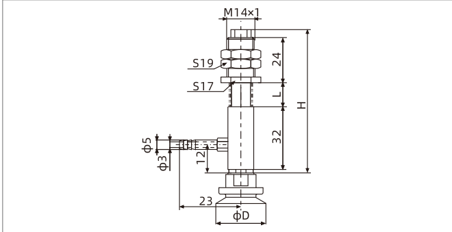
SPA25-50 水平方向 - 宝塔接头
