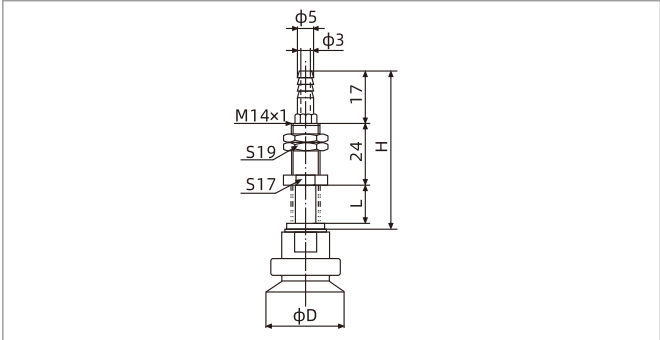
SPA25-50 垂直方向 - 宝塔接头
