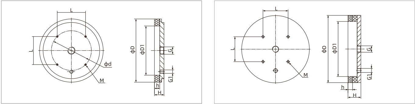
SOP40-180
