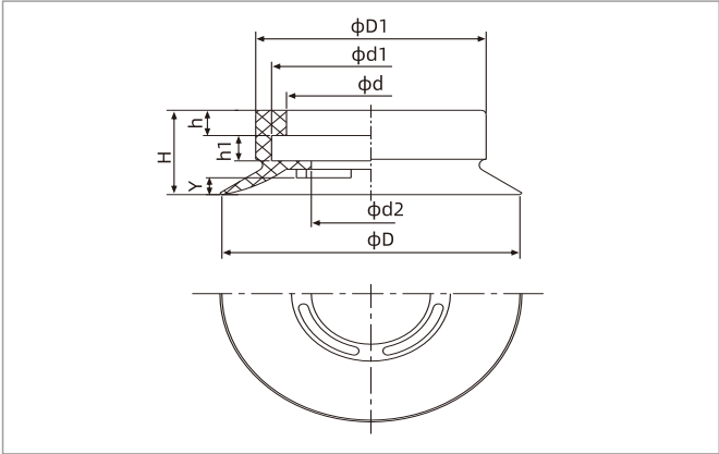
SPU30-100 ◇ 注：尺寸公差符合GB/T3672.1-2002-1 M3橡胶制品尺寸公差标准中的要求。
